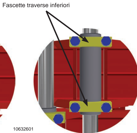
Dettaglio A Passaggio n. 4
