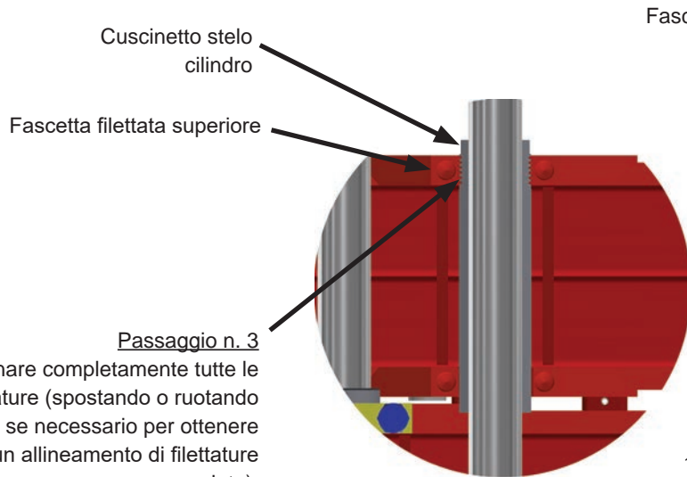
Dettaglio A Passaggio n. 3
